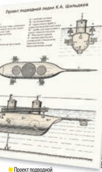
■ Проект подводной лодки Карла Шильдера
